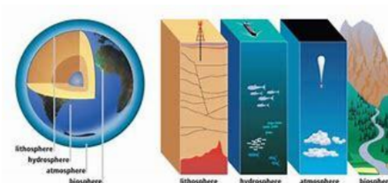
Gambar 1.8 Geosfer
