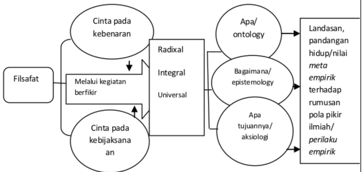
Gambar 1: Karakteristik Filsafat
