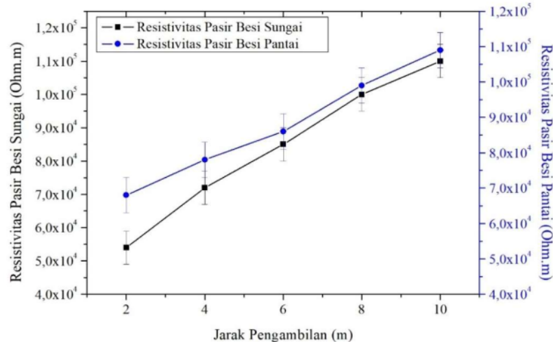
Gambar 2 Grafik perbandingan resistivitas pasir besi sungai dan pantai
